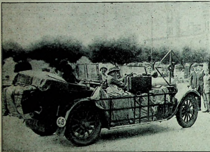
De opstelling van toestel en raamantenne.
